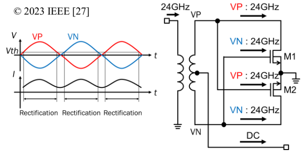
Fig. 7 Rectification operation in rectifier.
